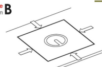
Edelstahl Rahmen zum flächenbündigen Einbau Stainless steel support frame for flush installation
